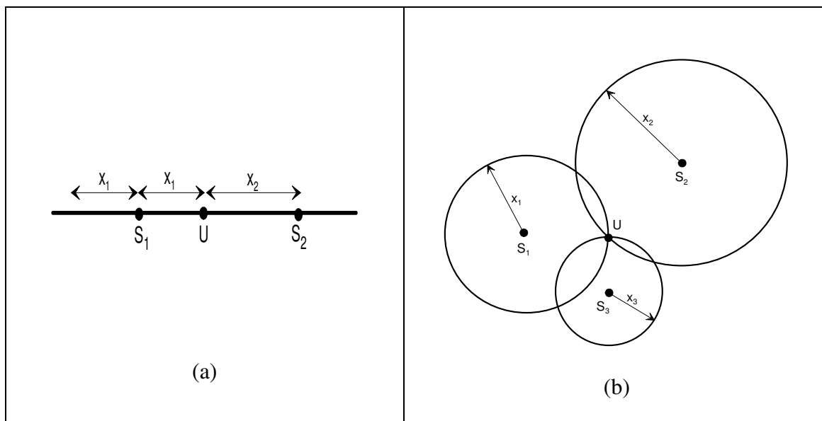
Fig. 4.3 – Posicionamento (a) unidimensional e (b) bidimensional de um usuário U .
