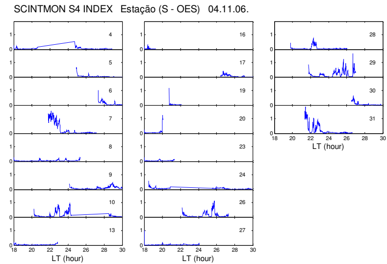
Fig. 6.3 - Os diversos painéis mostram os valores do índice S_4 , calculado para os sinais mostrados na Figura 6.2. Valores de S_4 acima de 0.2 estão associados à irregularidades.
